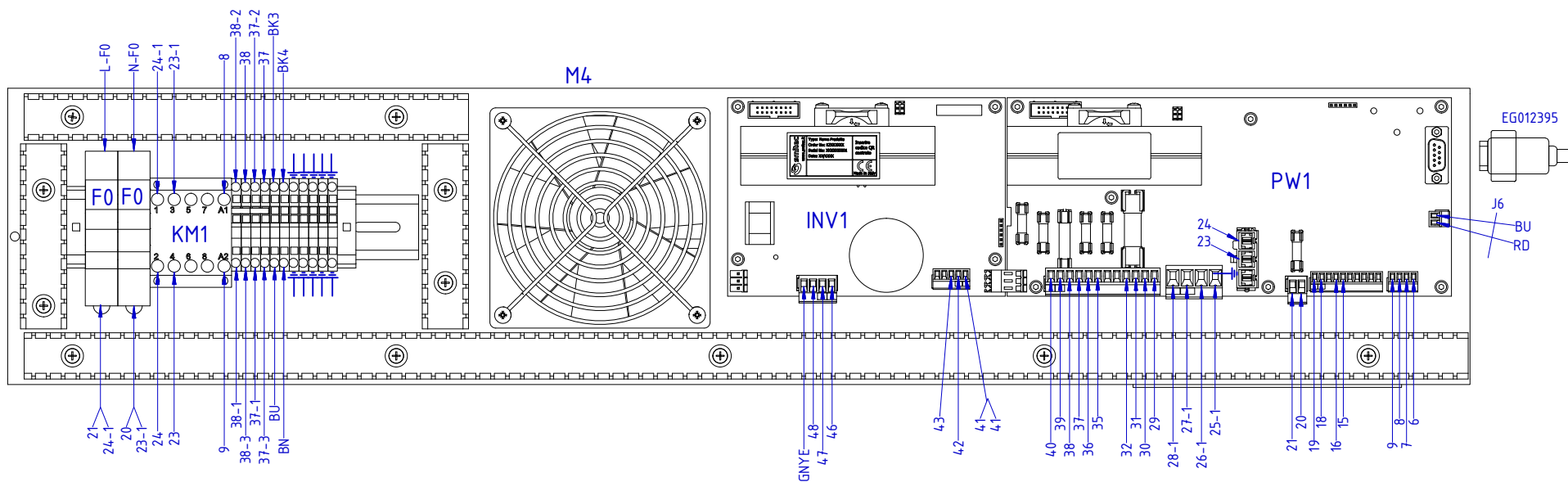
VISTA TRASFORMATORE
