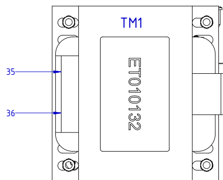
VISTA TRASFORMATORE
